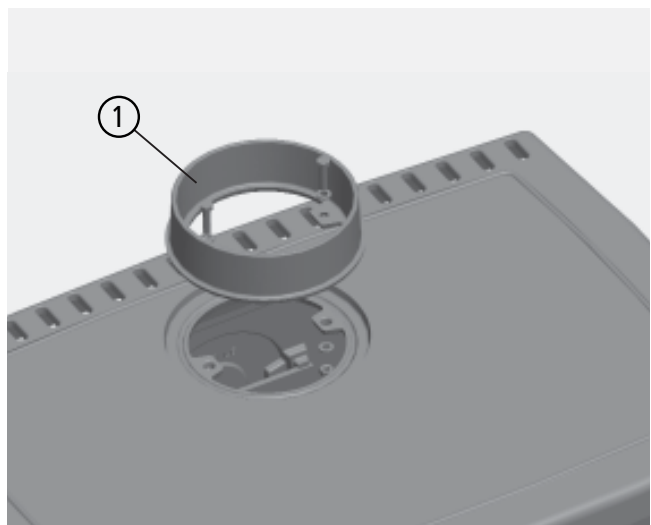
Abb. 3.2 Abgasstutzen auf der Deckplatte montieren
