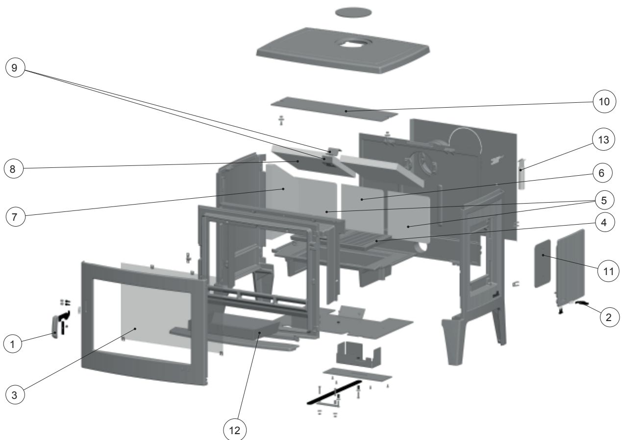
Abb. 5.1 Ersatzteilübersicht für ALLEGRA
