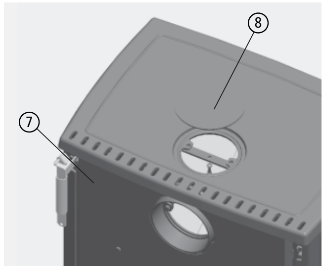
Abb. 3.5 Rückwandblech und Blinddeckel montieren
