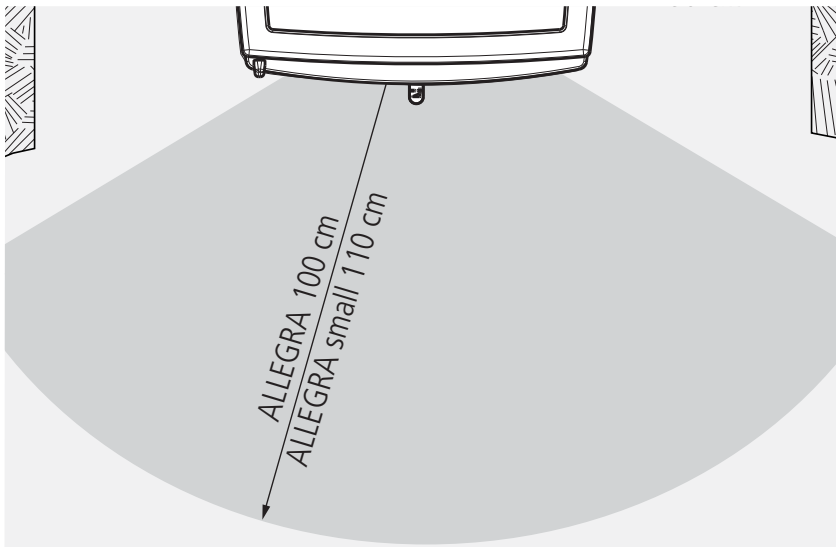
Abb. 1.4 Mindestabstände im Bereich der Sichtfenstertür
