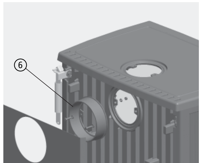
Abb. 3.4 Abgasstutzen an der Rückwand montieren
