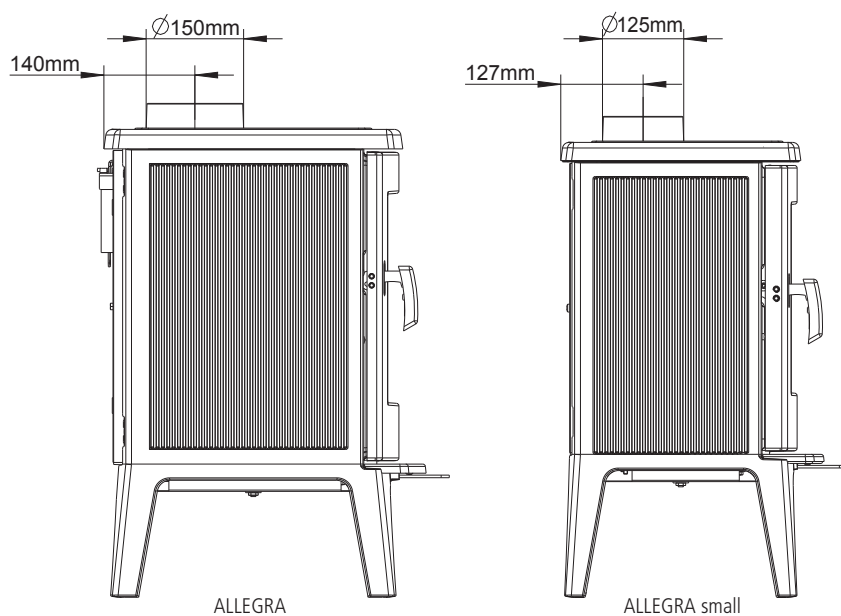
Abb. 3.6 Abgasanschlussmaße bei Anschlussstutzen nach oben
