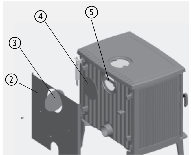
Abb. 3.3 Rückwandblech und Blinddeckel demontieren
