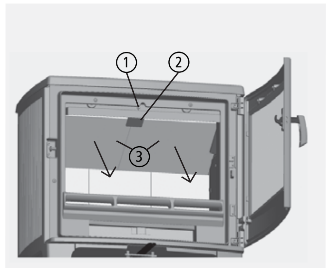
Abb. 4.14 Entnahme der Umlenplatten
