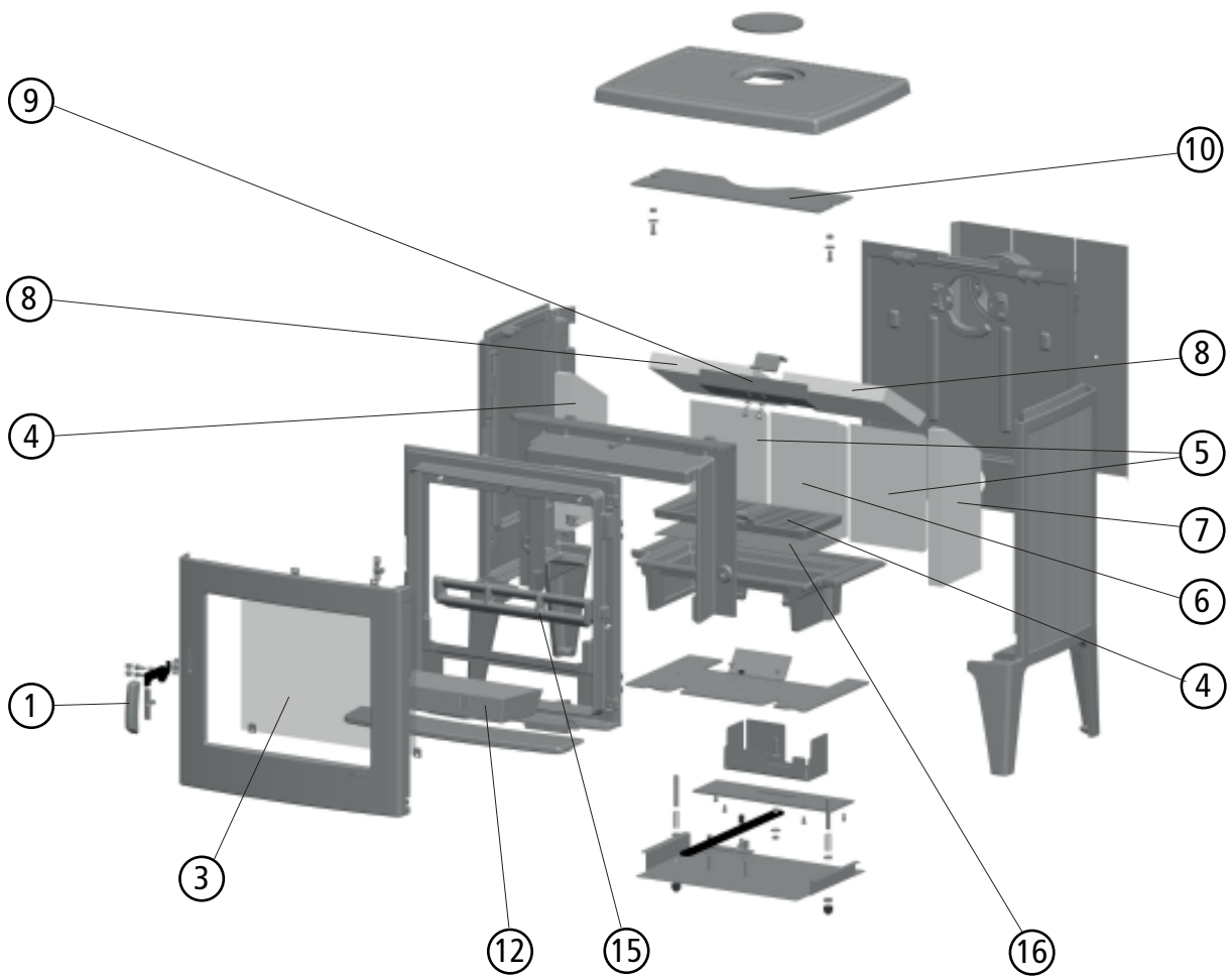
Abb. 5.2 Ersatzteilübersicht für ALLEGRA small
