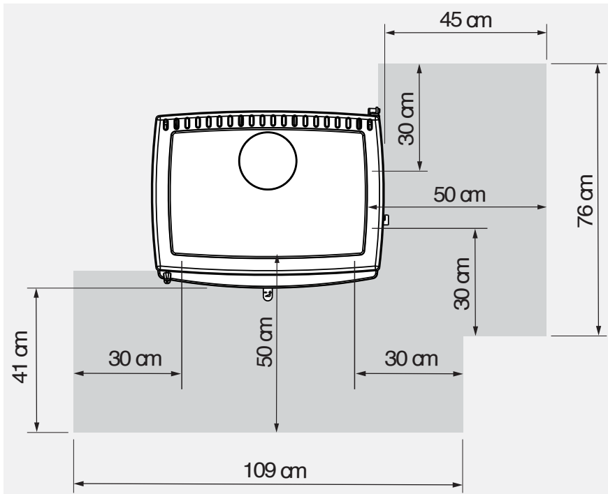
Abb. 1.2 Nicht brennbarer Belag vor den Feuerraumöffnungen beim ALLEGRA
