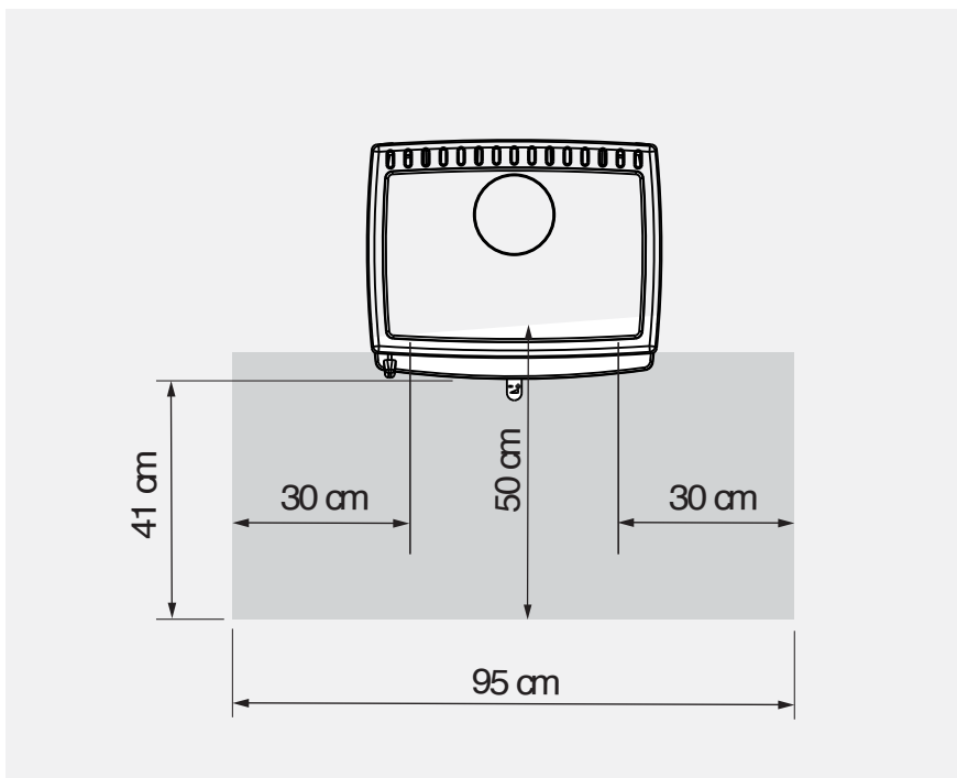
Abb. 1.3 Nicht brennbarer Belag vor den Feuerraumöffnungen beim ALLEGRA small
