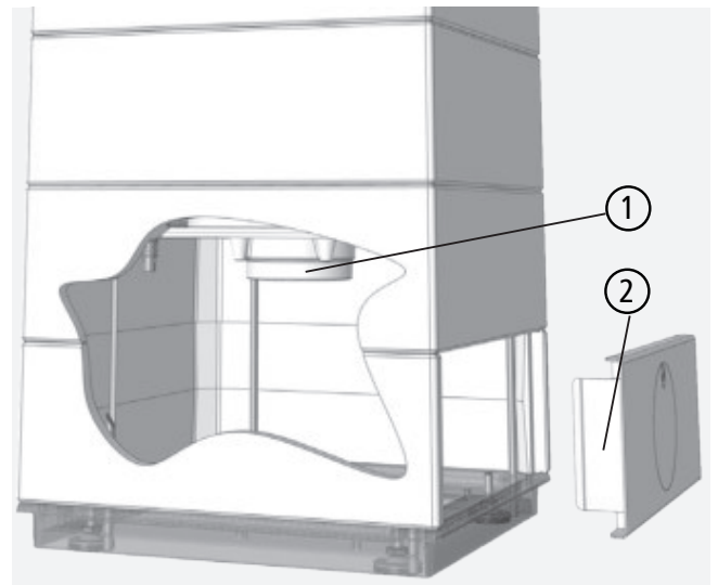
Abb. 3.1 Verbrennungsluftstutzen
