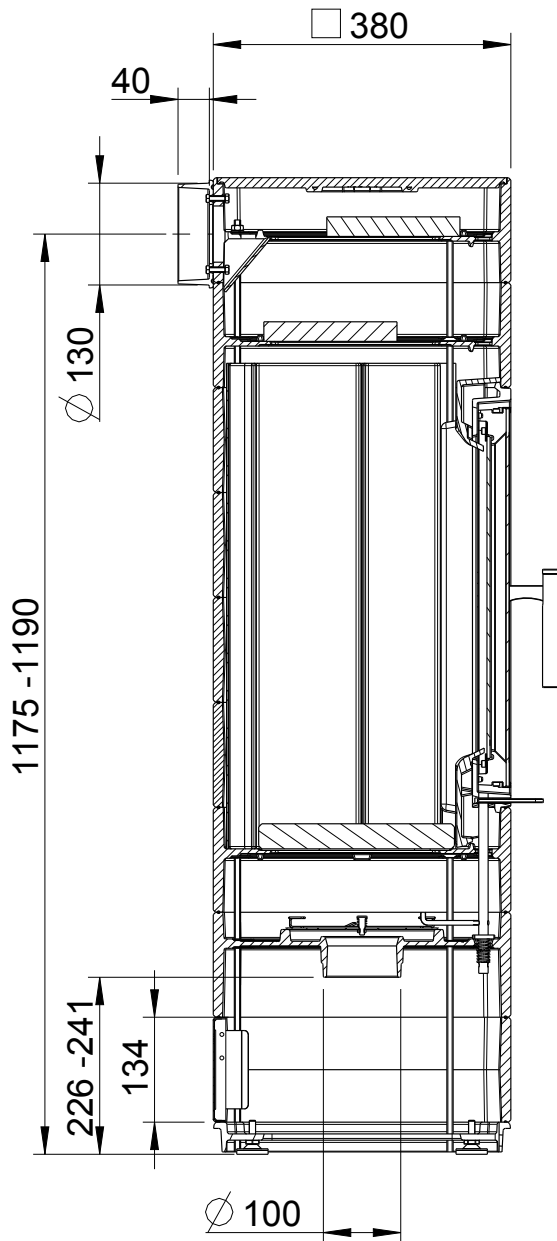
Abb. 3.12 Abgasanschluss, Maße bei Anschlussstutzen nach hinten
