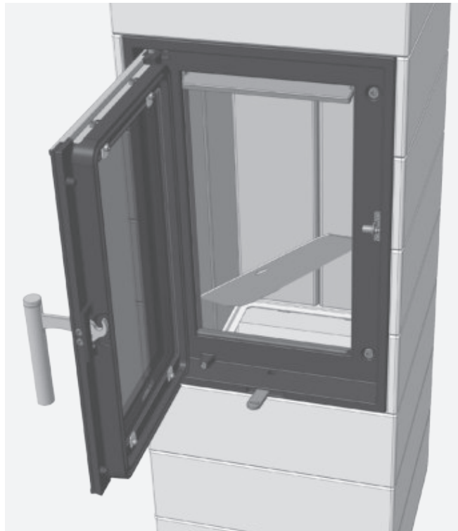
Abb. 4.13 Entnehmen des Bodenblechs im Brennraum
