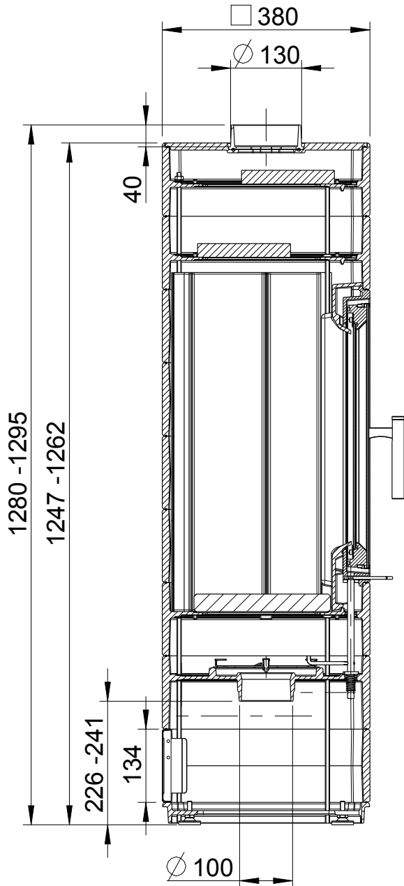
Abb. 3.11 Abgasanschluss, Maße bei Anschlussstutzen nach oben
