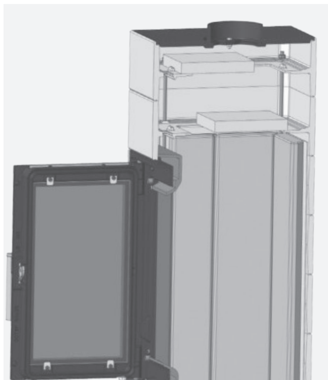
Abb. 4.14 Entnehmen des Bodenblechs im Brennraum
