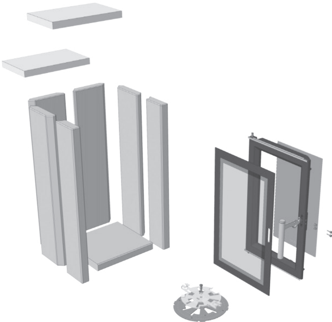
Abb. 8.1 Ersatzteilübersicht für CORNA
