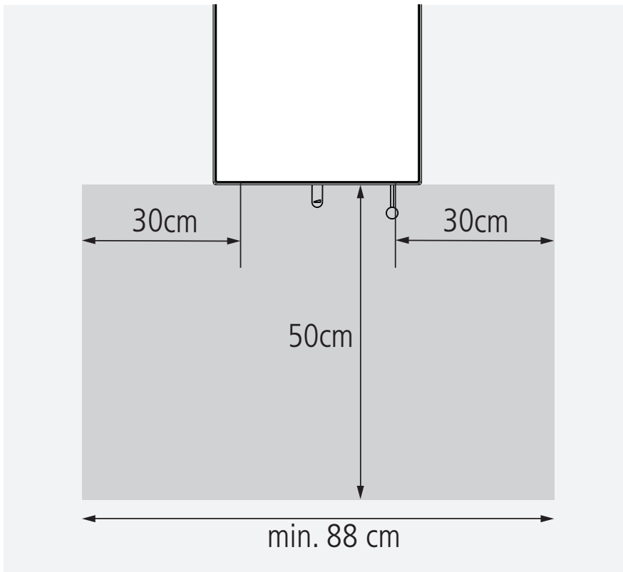
Abb. 1.2 Nicht brennbarer Belag vor den Feuerraumöffnungen
