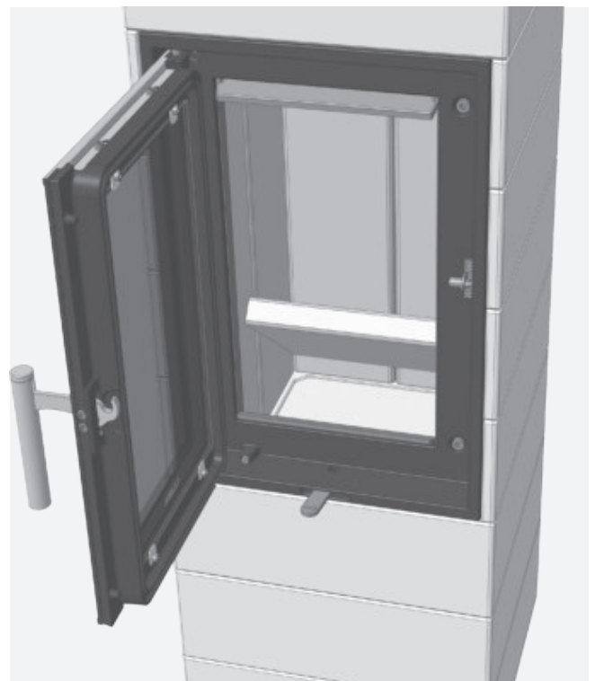
Abb. 4.12 Entnehmen des Bodensteins im Brennraum
