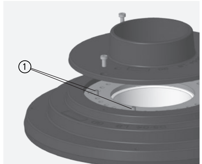
Abb. 3.8 Madenschrauben zur Einstellung des Drehwinkels
