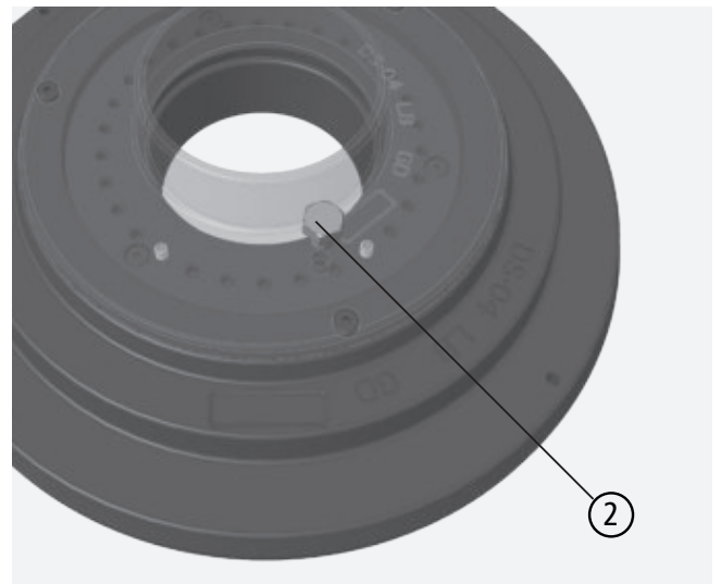
Abb. 3.9 Schraube für den Drehanschlag
