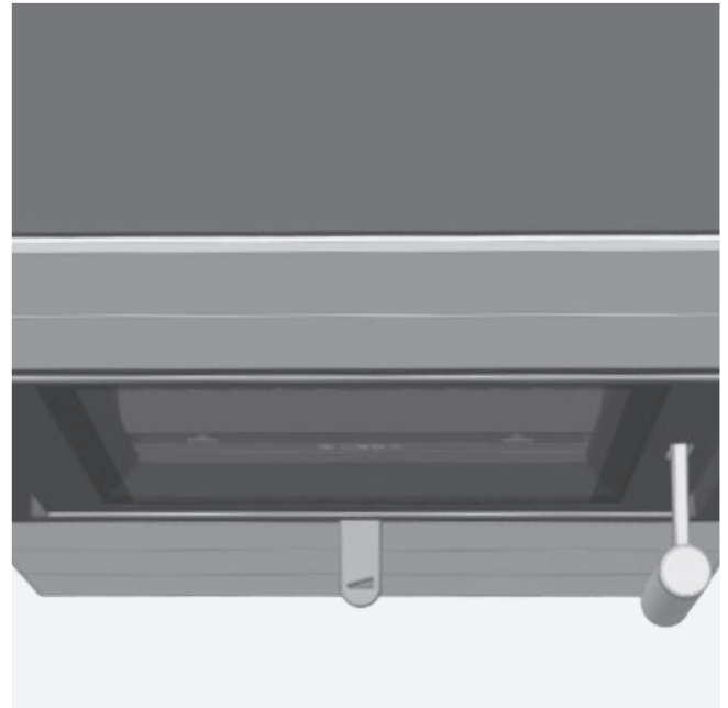
Abb. 4.9 Verbrennungslufthebel mittig, Verbrennungsluft auf Nennwärmeleistung
