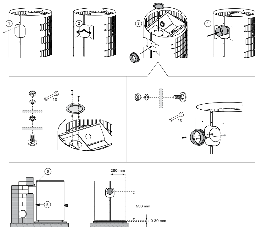
9. attēls. Pirts sildītāja savienošana ar mūra dūmvadu caur aizsmugurējo atvērumu.
