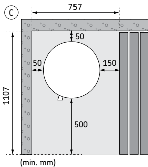
Abbildung 6. Sicherheitsabstände
