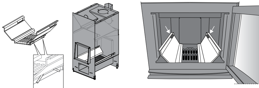
Abbildung 2. Verbrennungsluftleitbleche
