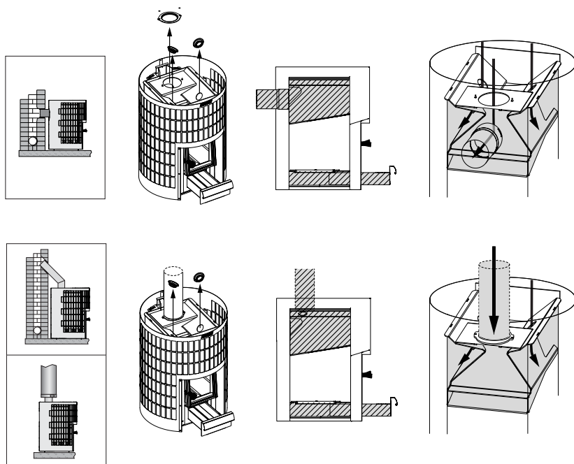
Рисунок 16. Чистка каменки
