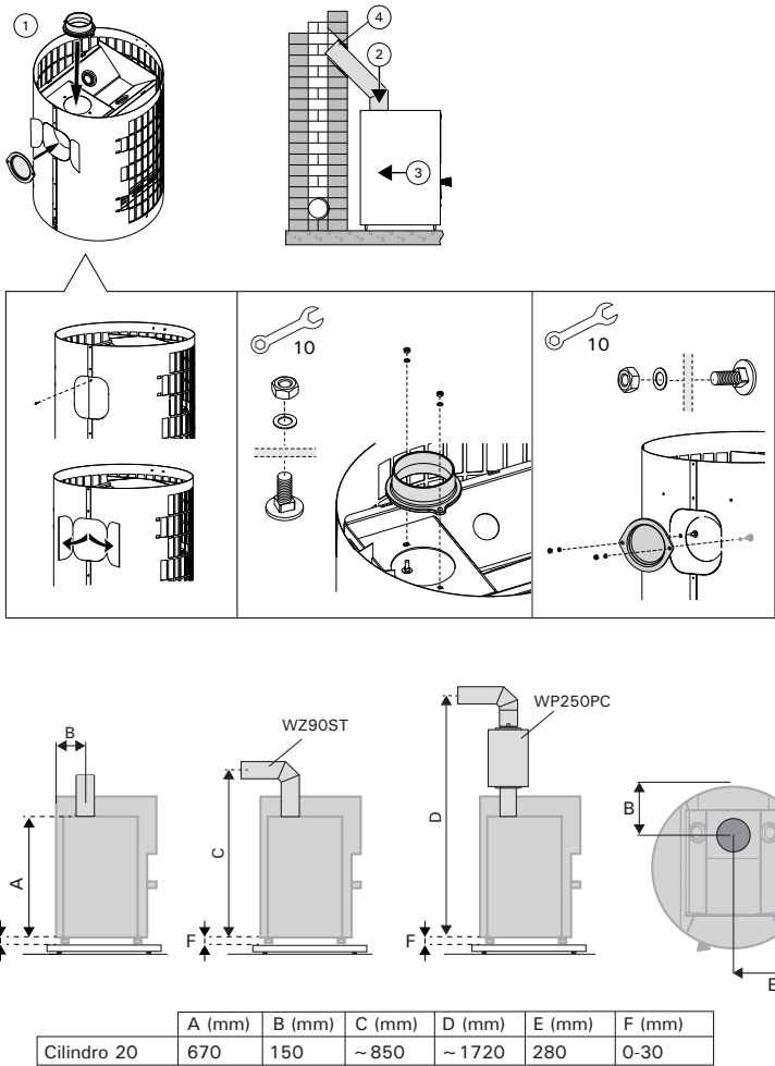
Abbildung 10. Anschluss des Saunaofens an einen gemauerten Rauchabzug durch die obere Öffnung
