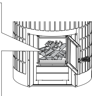
15. attēls. Pirts sildītāja sakarsēšana
