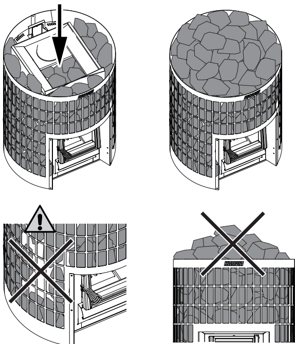
Abbildung 14. Befüllung der Steinkammer
